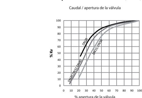
Kv en función de la apertura de la válvula. (G 4.3)
